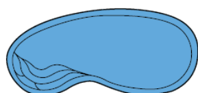
Modèle 75 Dimensions 3,80m x 7,75m Fond en pente 1,33m - 1,60m
