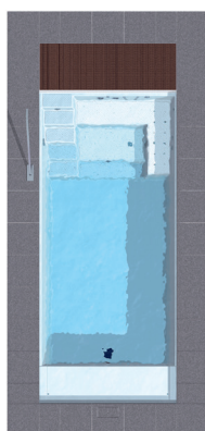
MODENA 550 S&F 2,7 x 5,5 x 1,5 m
